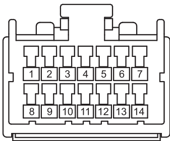
RF09a 天窗开关线束连接器（海外）
