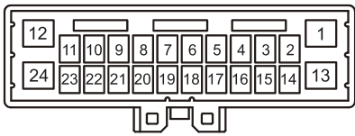
RF07 天窗模块线束连接器
