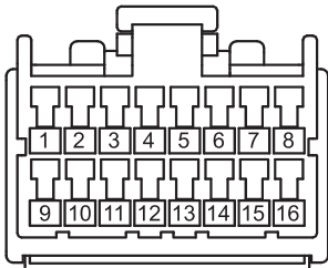
RF12 行车记录仪线束连接器
