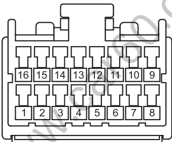
RF09 天窗开关线束连接器
