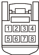
RF14 降噪模块线束连接器
