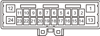
RF06 乘员侧安全气囊线束连接器
