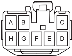
RF09 天窗开关线束连接器
