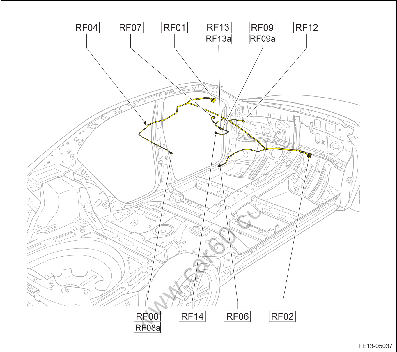
顶棚线束布置图
